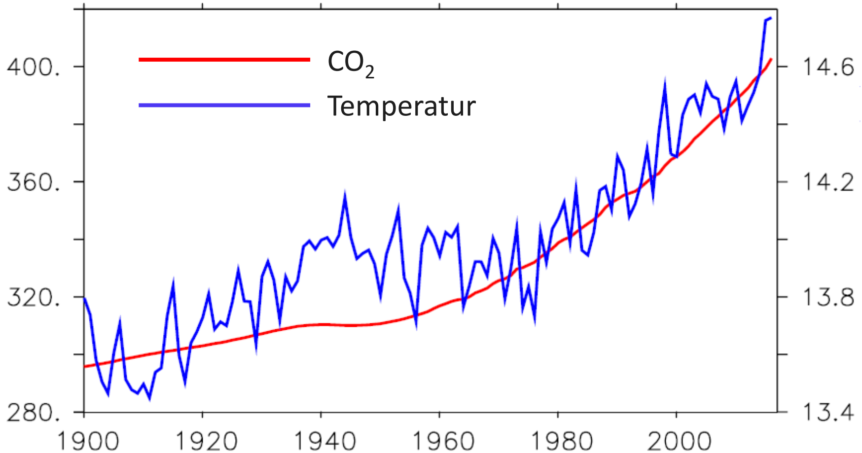
Globale Mitteltemperatur und der CO 2 -Gehalt der Luft
